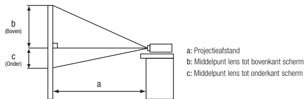
Eenheid: mm
